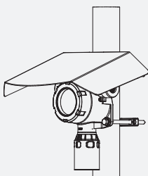
Sunshade/Deluge protection
