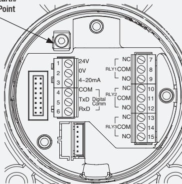
Terminal Module
